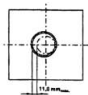
Juego máximo entre el dispositivo de centrado y el tubo para una base no regulable
